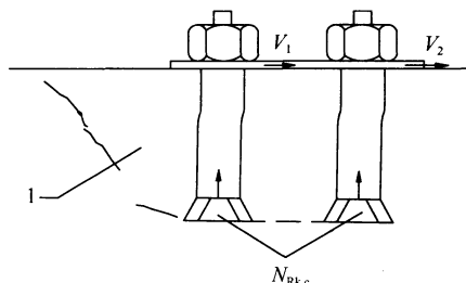
图 6.1.26 锚栓剪撬破坏示意
