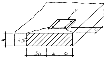
图 6.1.18-3 四栓受剪，位于构件角部示意
