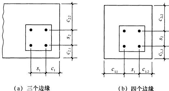
图 6.2.12 有多个边缘影响的群锚示意
