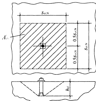
图 6.1.4 理想锥体破坏投影面积示意
