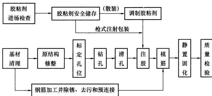
图 6 植筋施工工序示意
