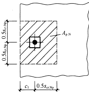
图 6.2.7-1 单栓受拉、靠近构件边缘时的计算面积示意
