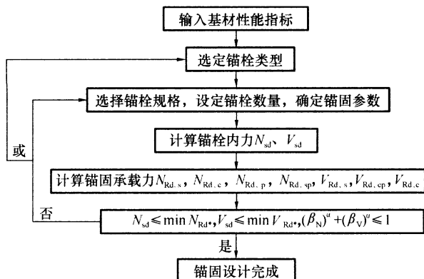
图 1 后锚固连接设计基本程序示意
