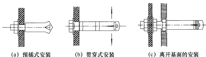
图 9.2.1 锚栓安装方式示意
