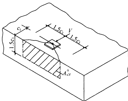
图 6.1.17 混凝土理想边缘破坏投影面积示意
