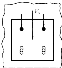
图 5.3.2 长槽孔处锚栓 不承担剪力示意
