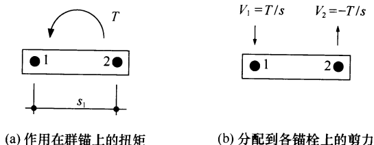
(a) 作用在群锚上的扭矩
