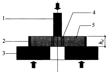
图 B.1.17 冲压测试示意
