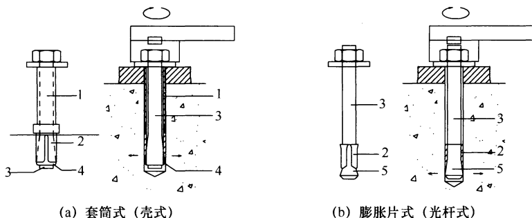
图 A.1.2-1 扭矩控制式膨胀型锚栓示意
