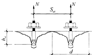
图 A. 2. 2 混凝土锥体 受拉破坏示意
