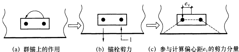
图 5.3.8-1 仅有扭矩作用示意
