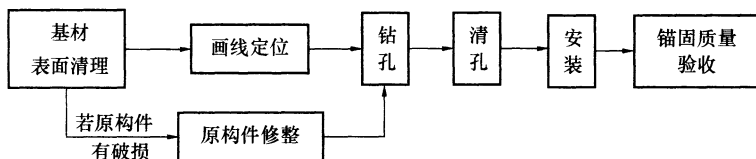
图 2 膨胀型锚栓施工工序示意
