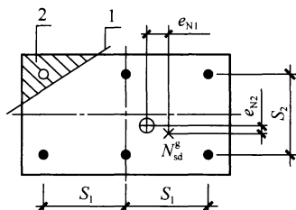
图 5.2.4-3 群锚双向偏心受拉示意
