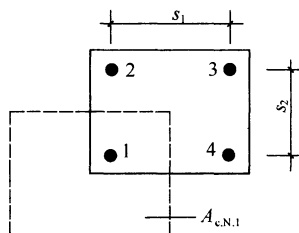
图 6.1.27-3 四栓，无边距影响示意
