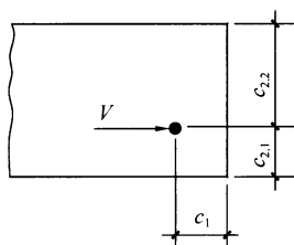
图 6.1.25 有多个边缘影响的锚栓示意
