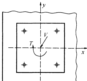
图 5.3.6 剪力和扭矩共同作用示意
