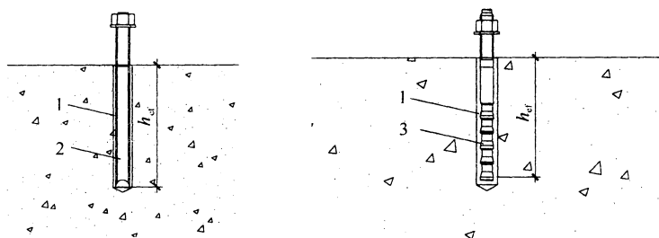
(a) 普通化学锚栓
