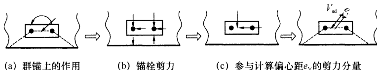
图 5.3.8-3 扭矩与剪力共同作用，
