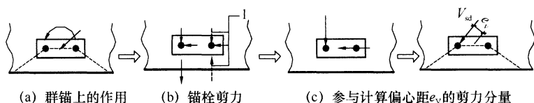
图 5.3.8-2 扭矩与剪力共同作用，
