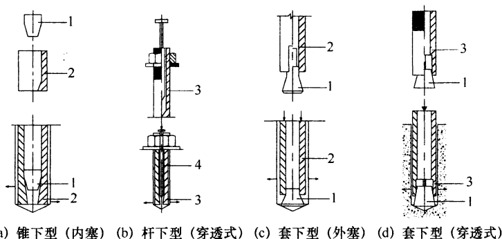
图 A. 1. 2-2 位移控制式膨胀型锚栓示意
