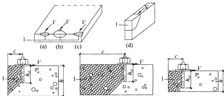
图 A. 2. 4 混凝土边缘楔形体受剪破坏示意
