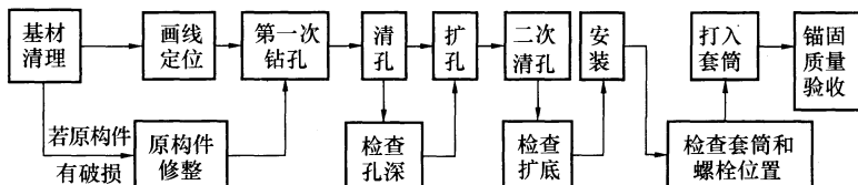
图 3 模扩底锚栓施工工序示意
