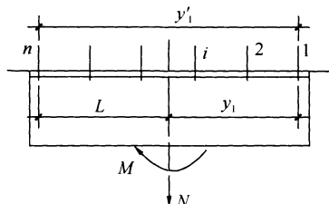
图 5.2.2 拉力和弯矩共同作用示意
