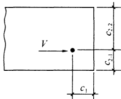
图 6.2.21 有多个边缘影响的锚栓示意
