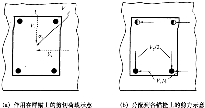
图 5.3.4 混凝土边缘破坏时锚栓受剪示意
