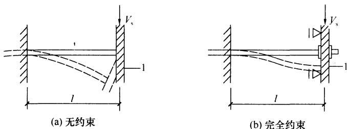
图 6.1.14-2 约束状况示意
