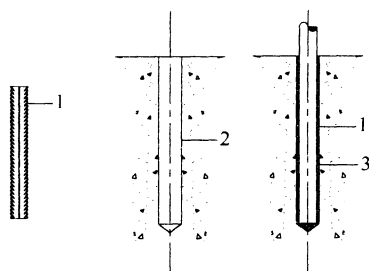
图 A.1.5 植筋示意
