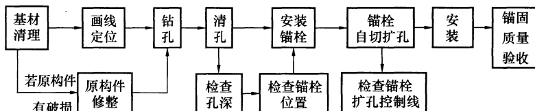
图 4 自扩底锚栓施工工序示意
