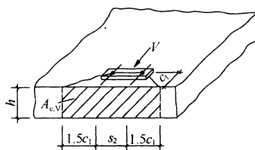
图 6.1.18-2 双栓受剪， 位于构件边缘示意
