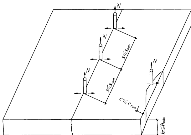
图 A. 2. 6 基材劈裂破坏示意
