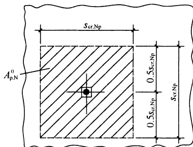
图 6.2.6 单个锚栓的影响面积 A_{p,N}^0 示意
