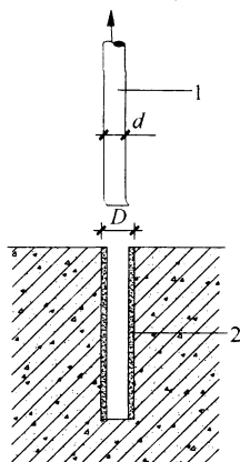
图 A.2.9 普通化学锚栓胶筋
