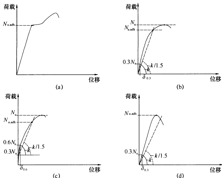
图 B.2.6 滑移荷载 N_{u,adh} 示意
