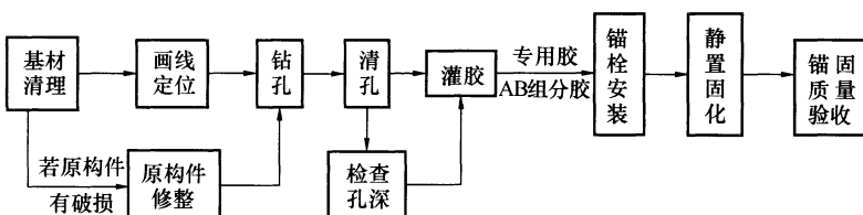
图 5 化学锚栓施工工序示意
