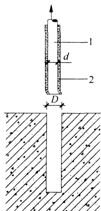
图 A.2.10 普通化学锚栓胶混
