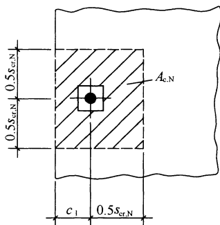
图 6.1.5-1 单栓受拉、靠近构件边缘时的计算面积示意
