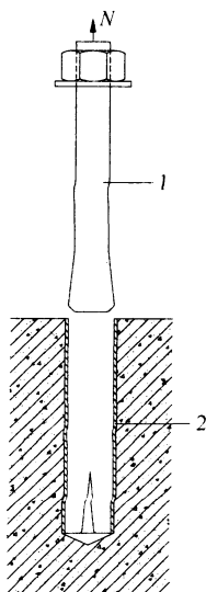
图 A.2.8 机械锚栓穿出破坏示意
