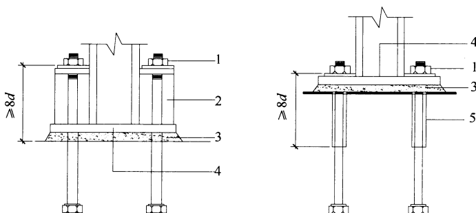
图 8.2.2 锚栓延性伸长段示意图
