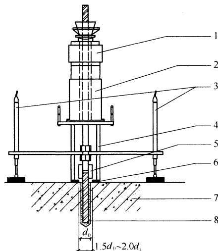
图 B.1.2 约束抗拉试验装置示意
