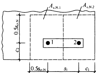
图 6.1.27-2 双栓，位于构件角部示意
