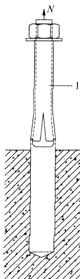
图 A.2.7 机械锚栓拔出破坏示意
