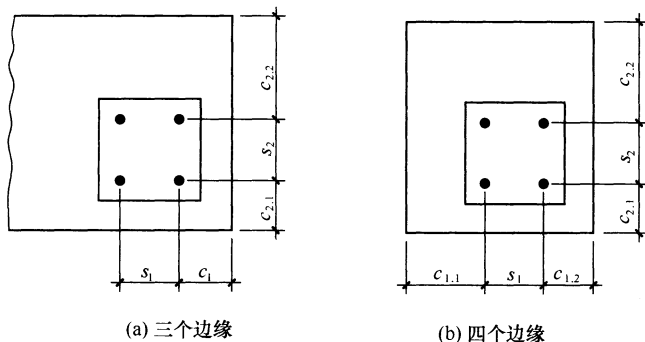
图 6.1.9 有多个边缘影响的群锚示意
