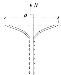
图 A. 2. 3 混合型 受拉破坏示意
