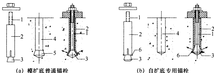
图 A. 1. 3 扩底型锚栓示意
