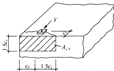
图 6.1.18-1 单栓受剪， 位于构件角部示意
